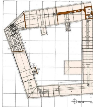
PŪDORYS KROVU
