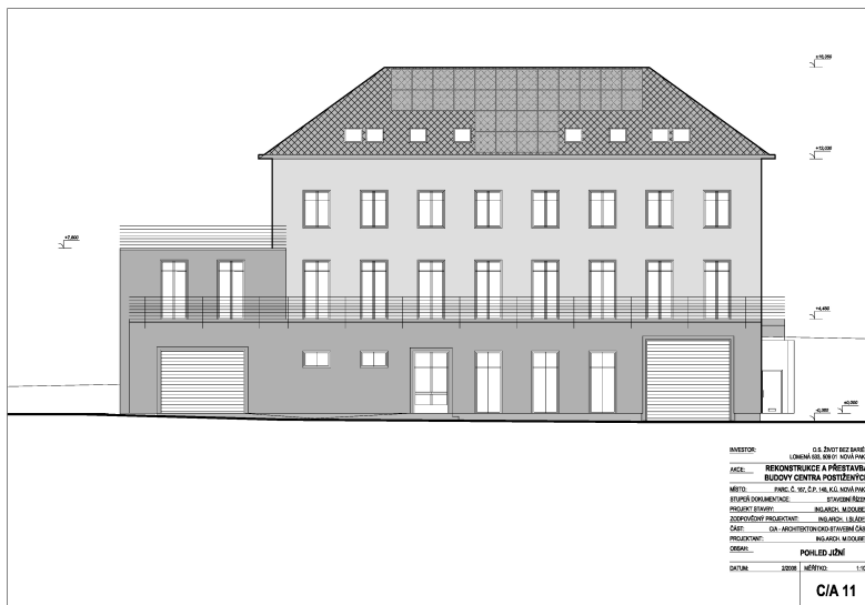
Pohled jižní
