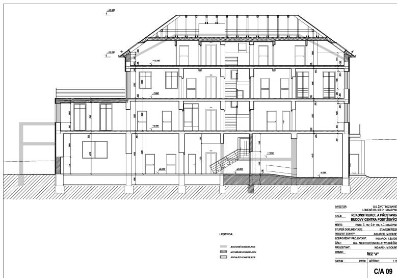
Řez "A"
