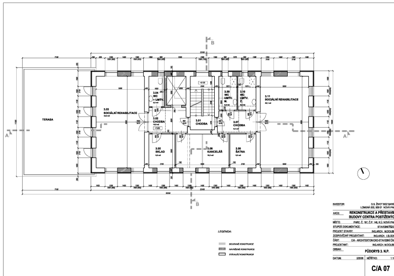
2. podlaží
